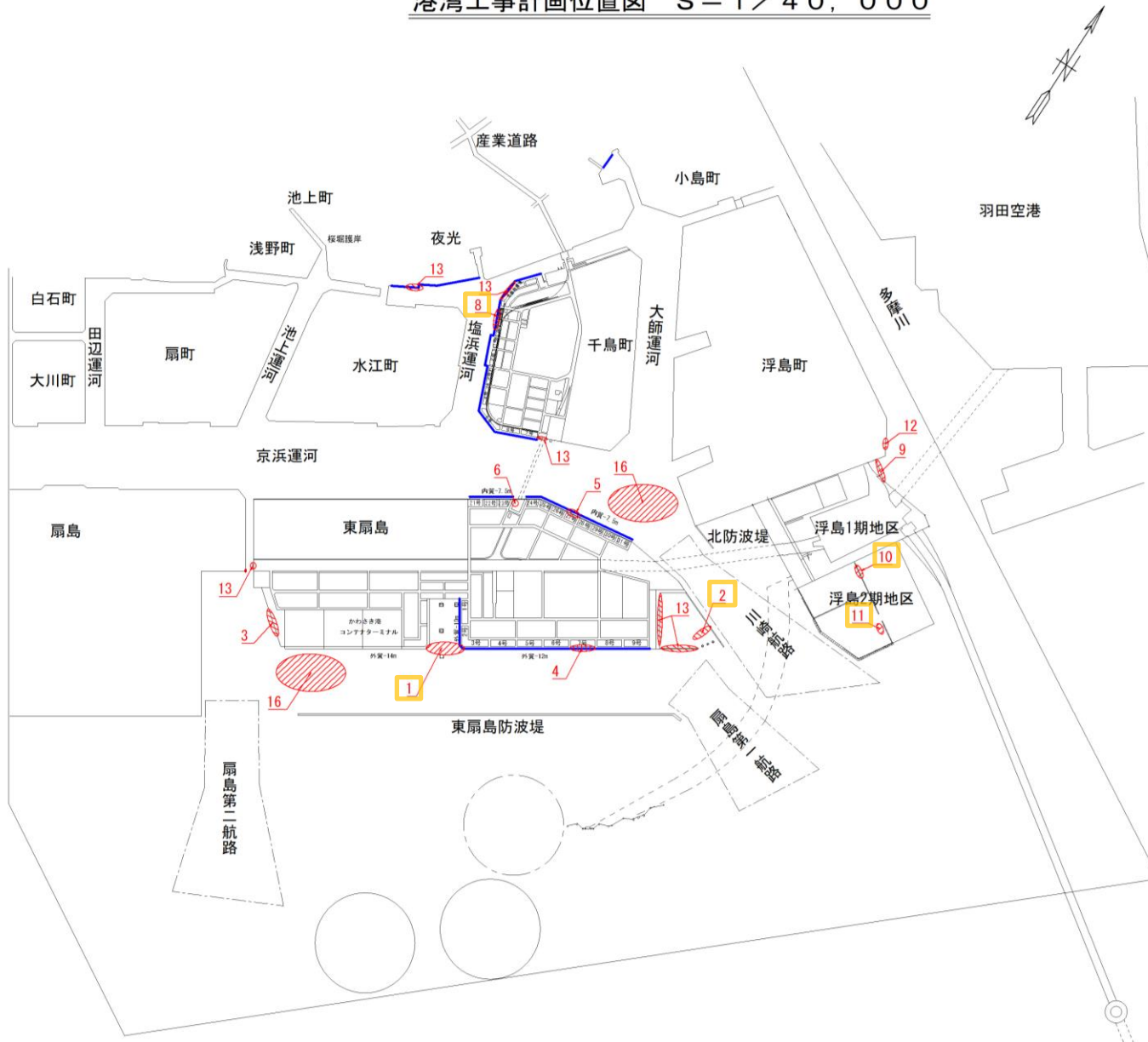
港湾工事計画位置図 S = 1 / 40, 000
